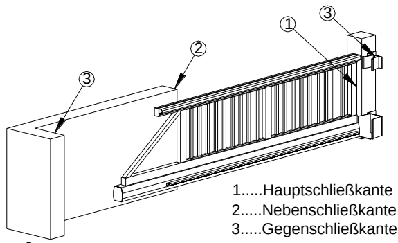
Abb. 1.3.1: Gefahrenbereiche
