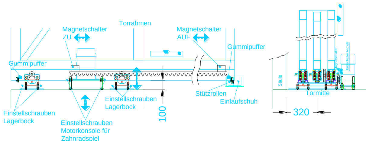
Abb. 7.2.1: Übersicht für Einstellungen (Darstellung bei geschlossener Torposition)
